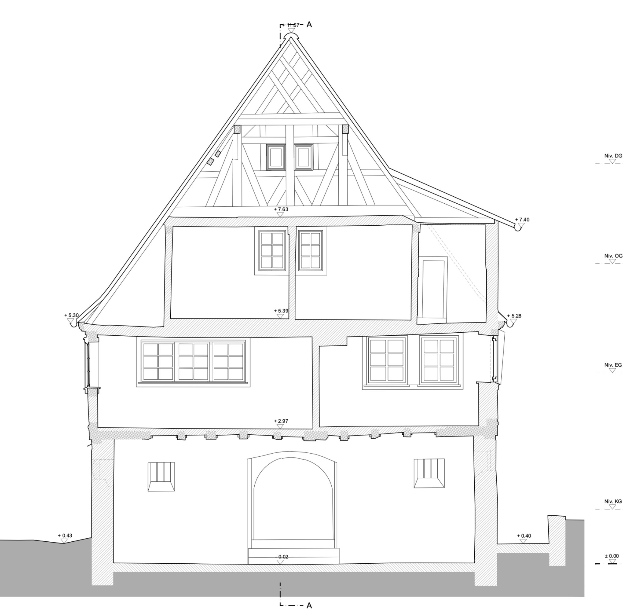
Schnitt DD
