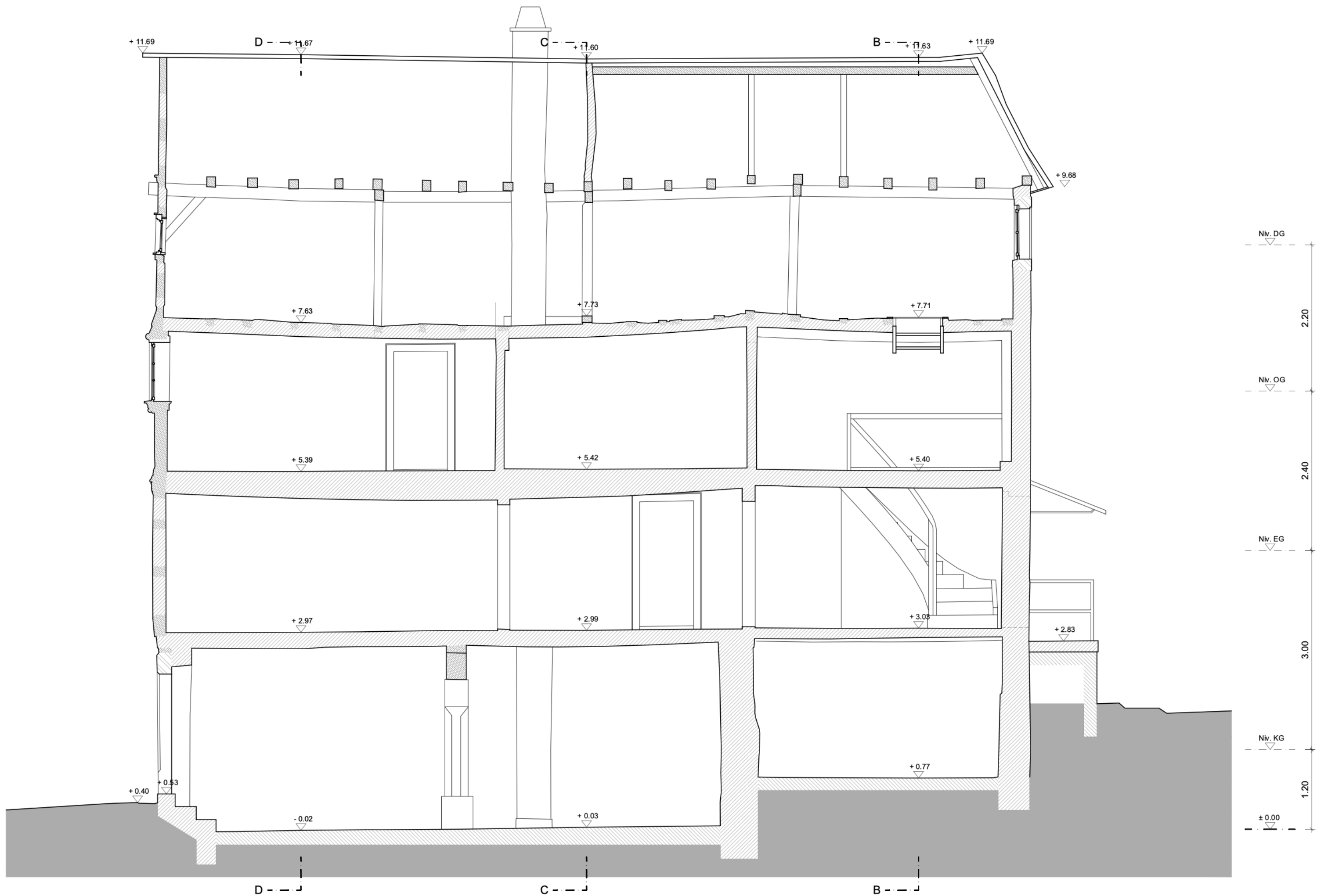
Schnitt AA
